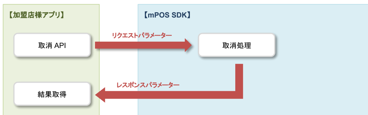
図 3 返金処理フロー
